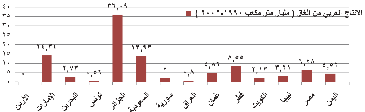
الشكل (١٦) إنتاج الغاز في الدول العربية
