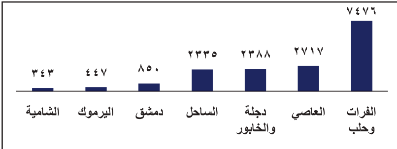
الشكل (٣) الموارد المائية في سورية حسب الأحواض (مليون م ٣ /سنة)
